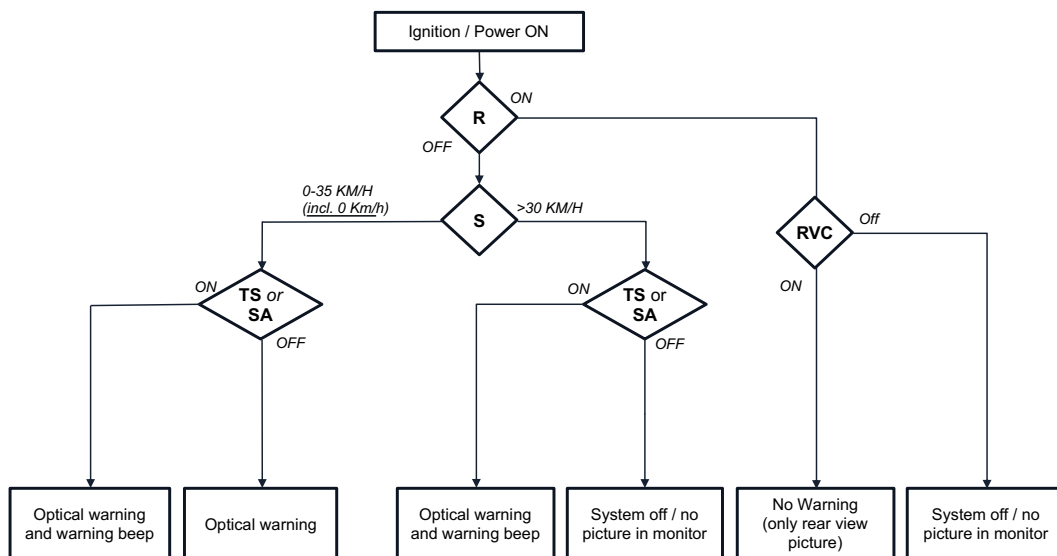
Abbildung 2: Software-Logik
